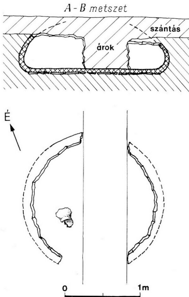
2. kép Esztergom-Diósvölgy. A kemence alap- és metszetrajza (1:25) Abb. 2. Esztergom-Diósvölgy. Grundriß- und Profilzeichnungen des Ofens (1:25)
